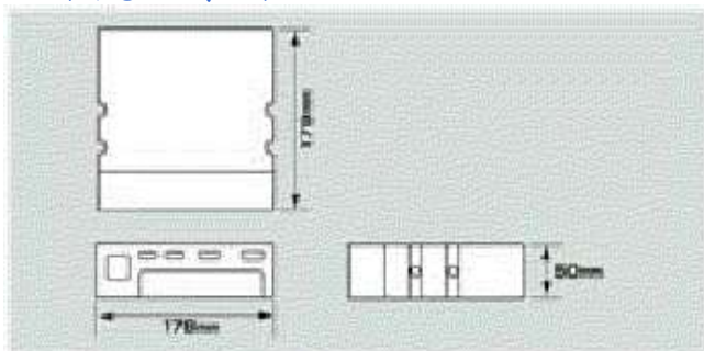
外觀尺寸圖
